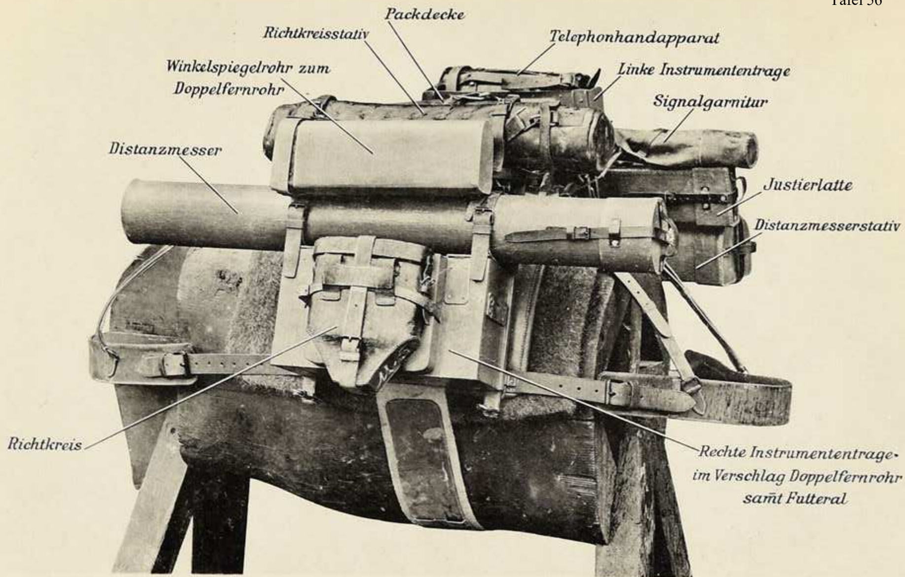
Instrumenten-Tragtier (Ansicht von rechts).
