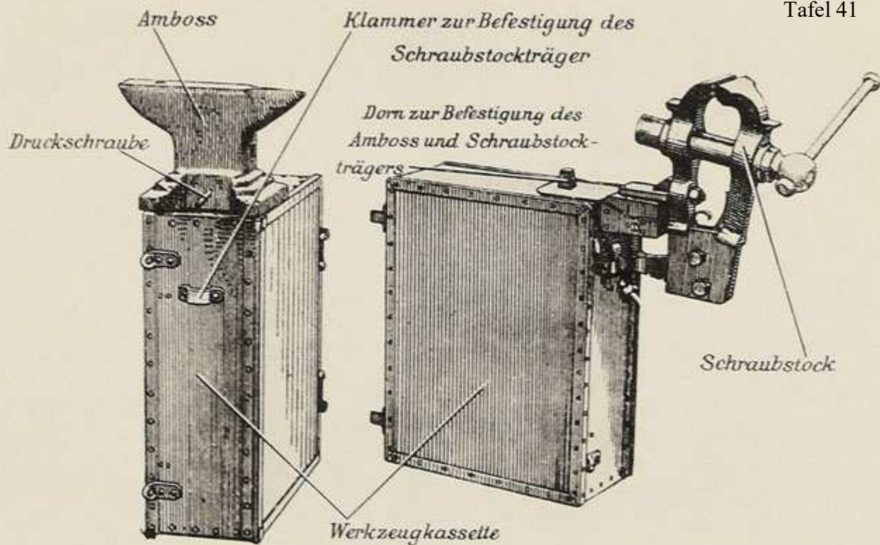
Werkzeugkassette mit Amboss, bezw. mit Schraubstock.
