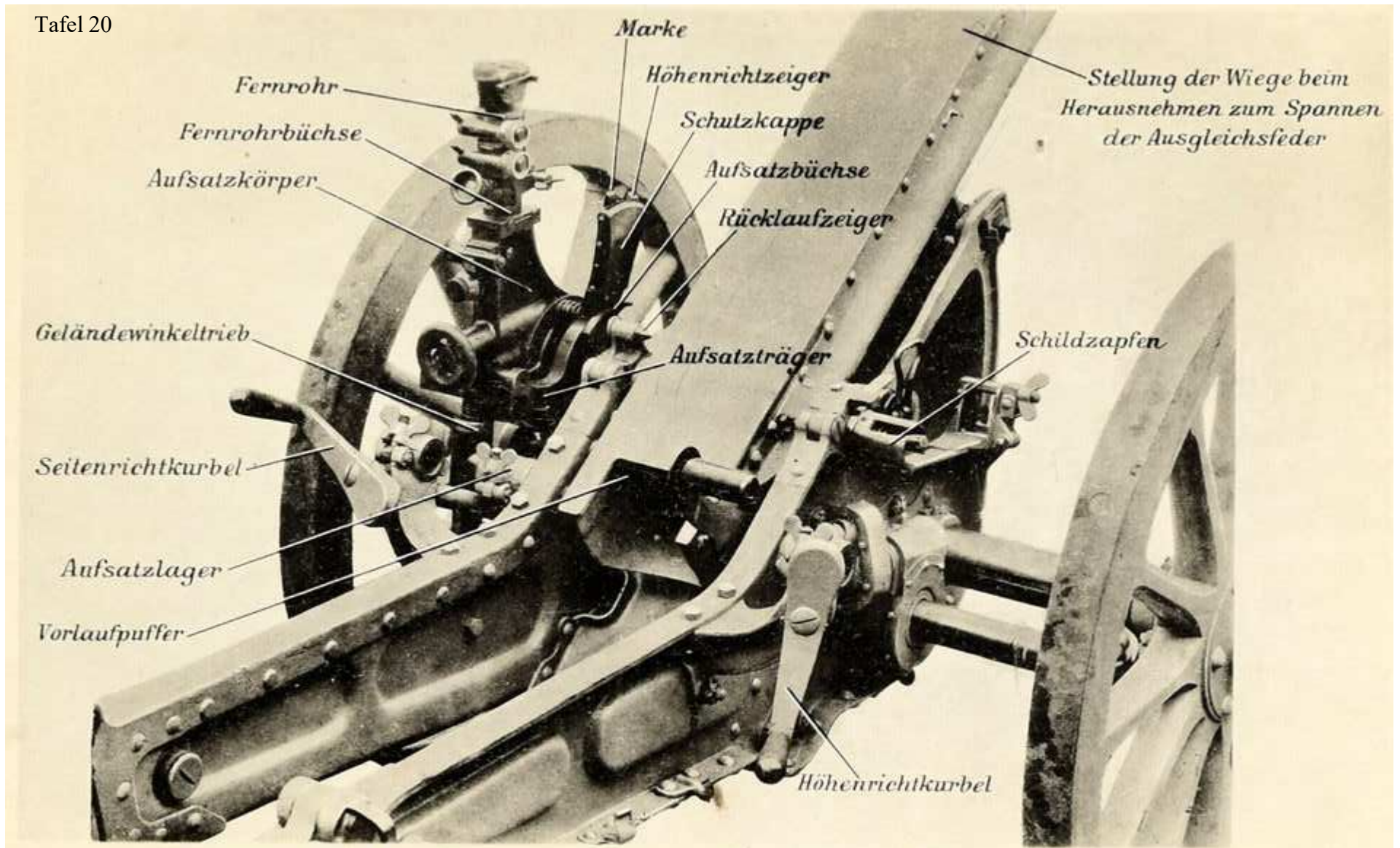
Geschütz (Ansicht von rechts rückwärts, Schutzschild und Rohr abgenommen).
