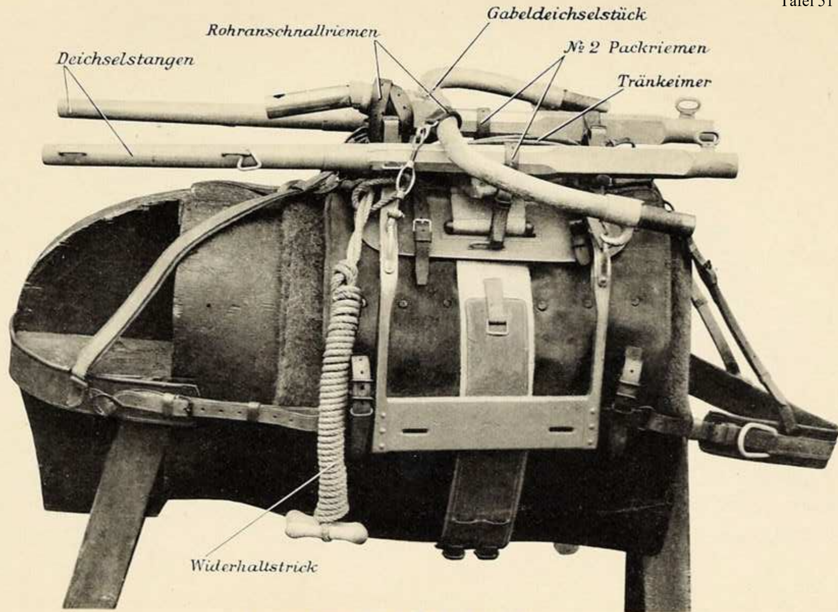
Auspackung der Gabeldeichsel.
