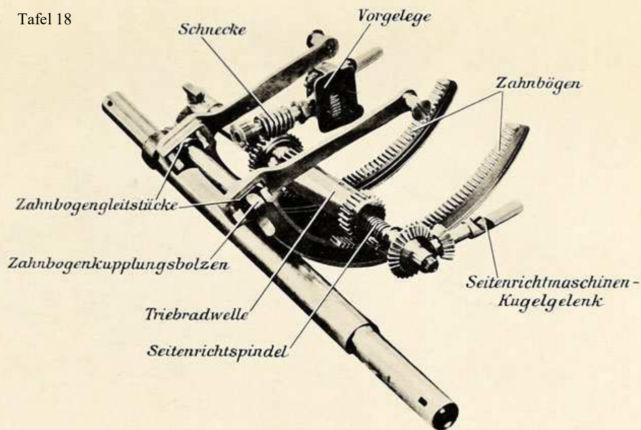
Schema der Richtmaschinen (Ansicht von links vorne).
