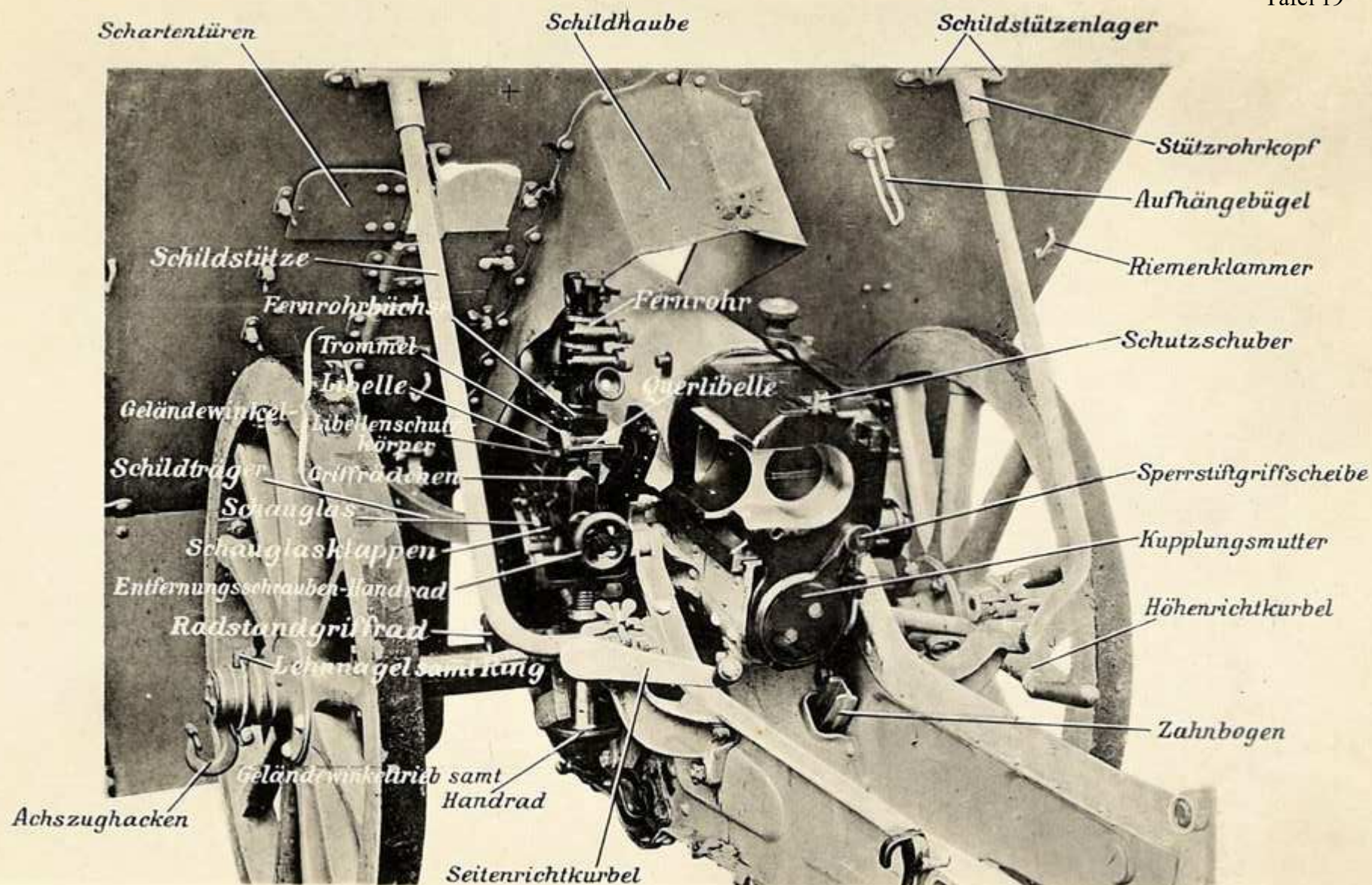
Geschütz (Ansicht von links rückwärts).
