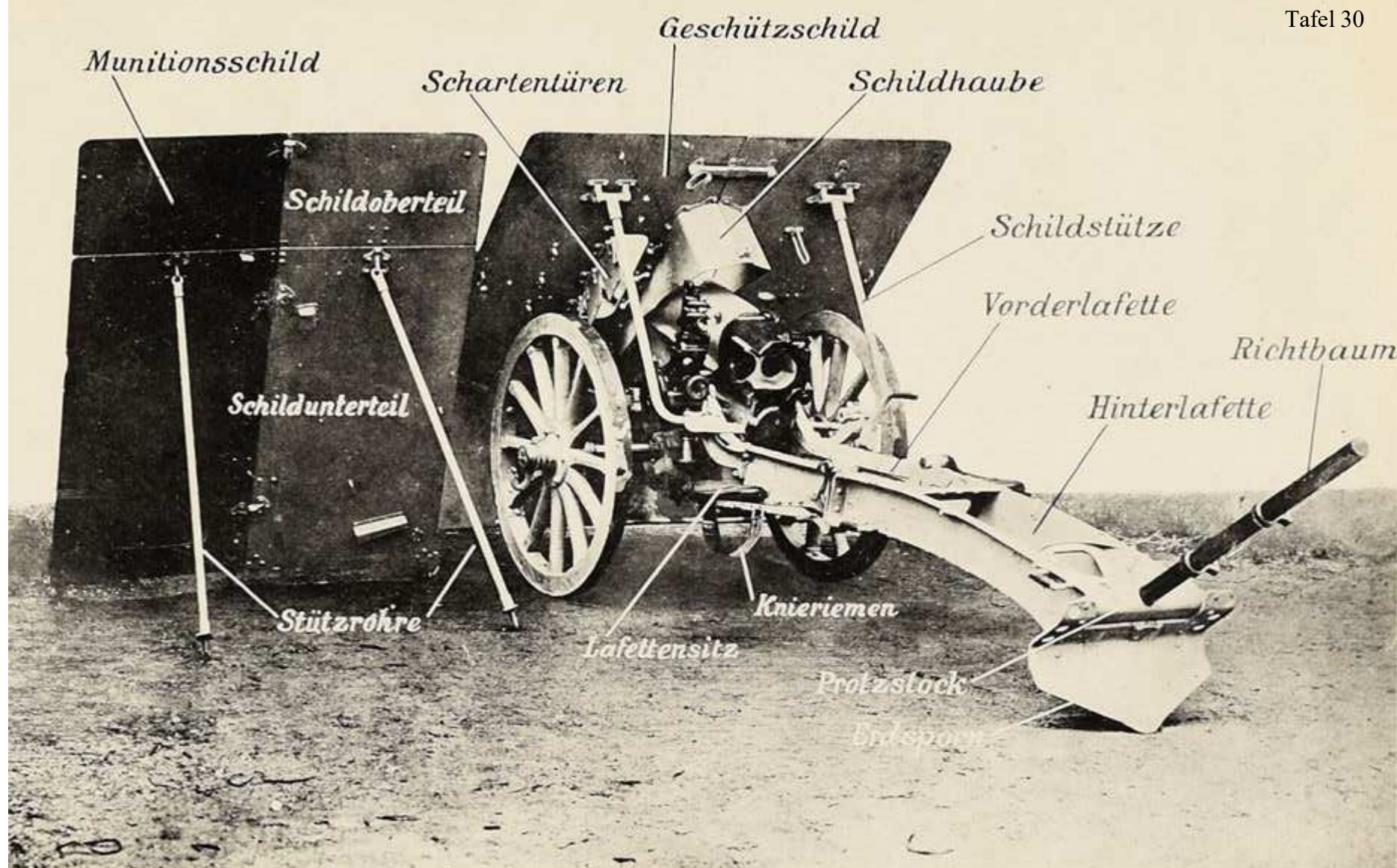
Geschütz samt Munitionsschild in Feuerstellung.
