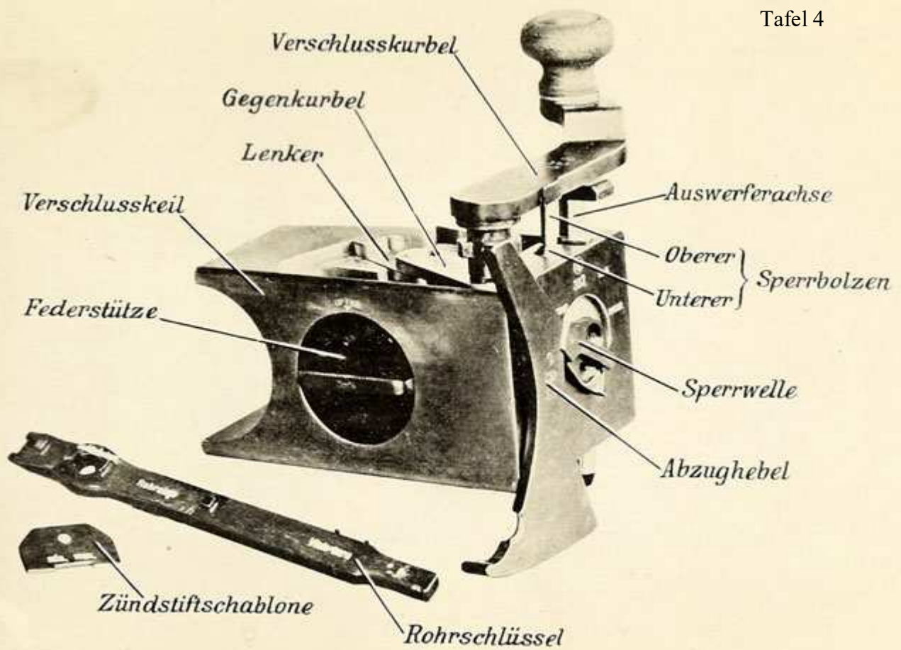
Verschluss (Ansicht von rechts rückwärts).
