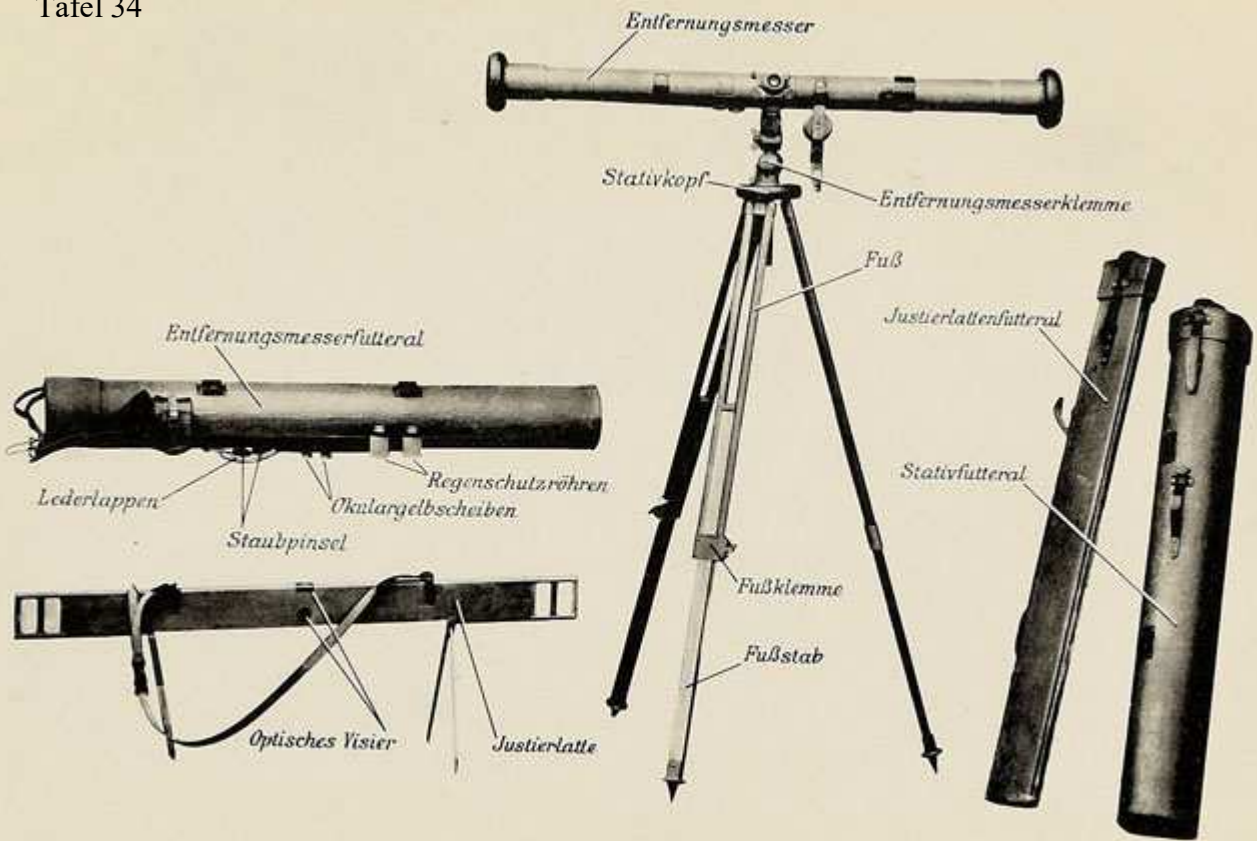
Entfernungsmesser samt Stativ und Behälter.
