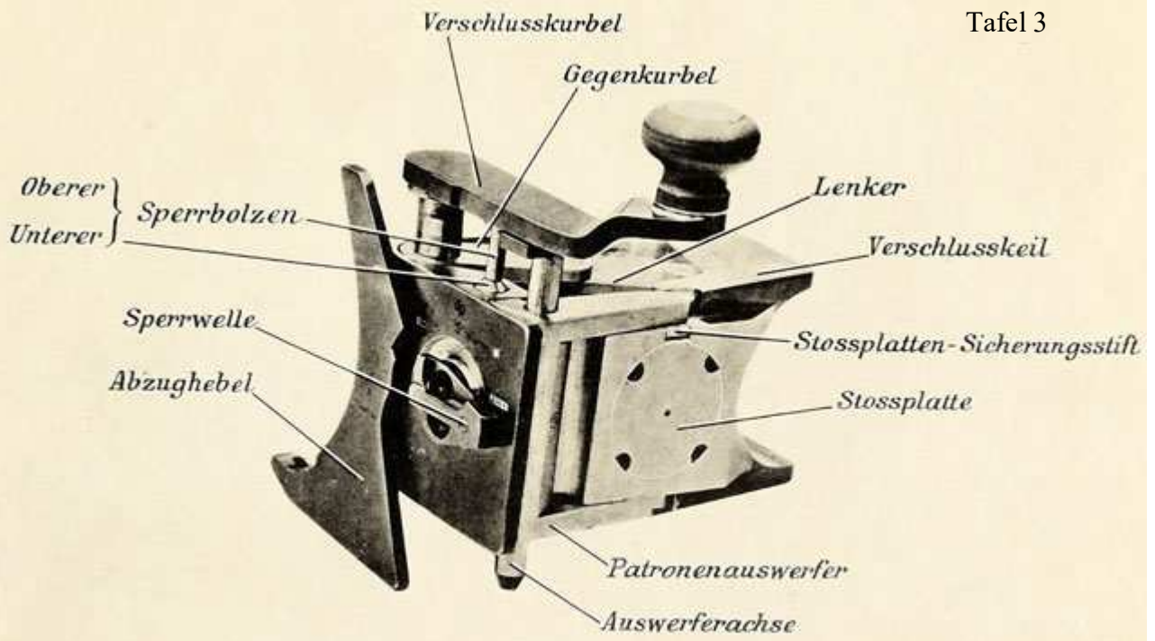
Verschluss (Ansicht von rechts vorne).
