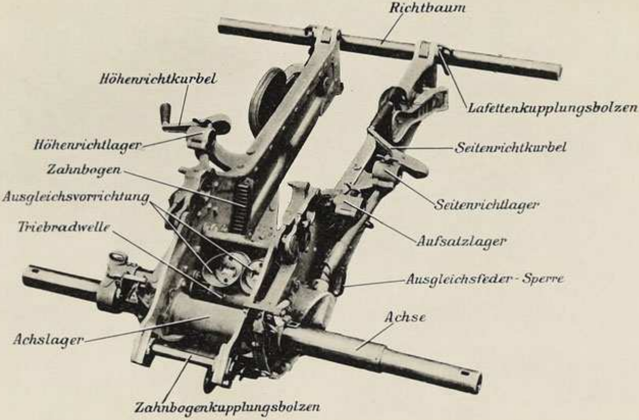
Vorderlafette mit Richtbaum.
