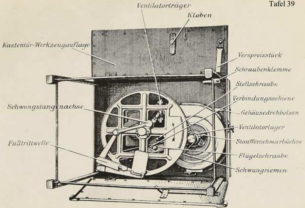
feldschmiede (halb zusammengelegt, Ansicht von unten).
