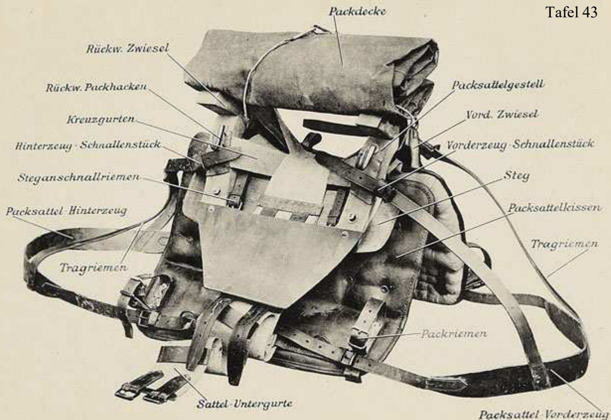
Munitions- und Bagage-Packsattel.
