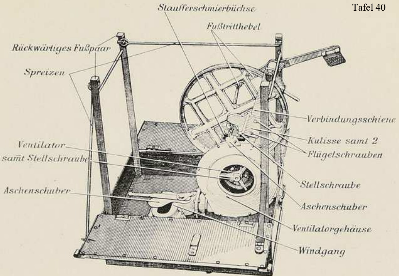
feldschmiede (Ansicht von unten).
